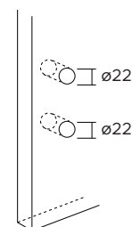
Bocchetta foro wc.
