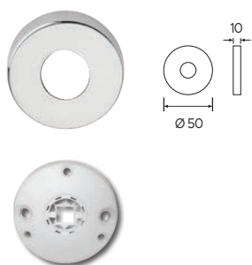
Rosetta. Sottorosetta in plastica con molla ambidestra. Rose. PVC under-construction.
