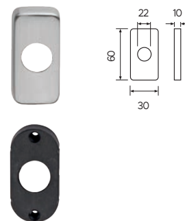
Bocchetta foro wc. Sottorosetta in plastica.
