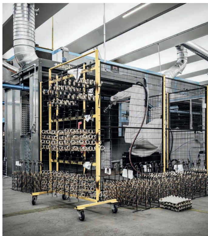
Impianto di verniciatura automatizzato. Automated painting system.
