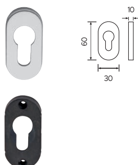
Bocchetta foro cilindro. Sottorosetta in plastica.
