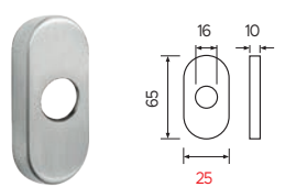
Rosetta DK stretto. Narrow DK cover.
