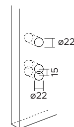
Bocchetta foro cilindro.
