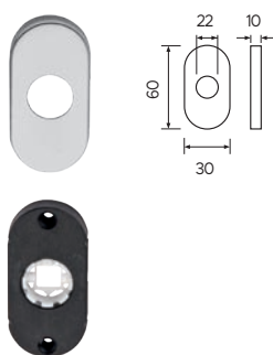
Rosetta. Sottorosetta in plastica.
